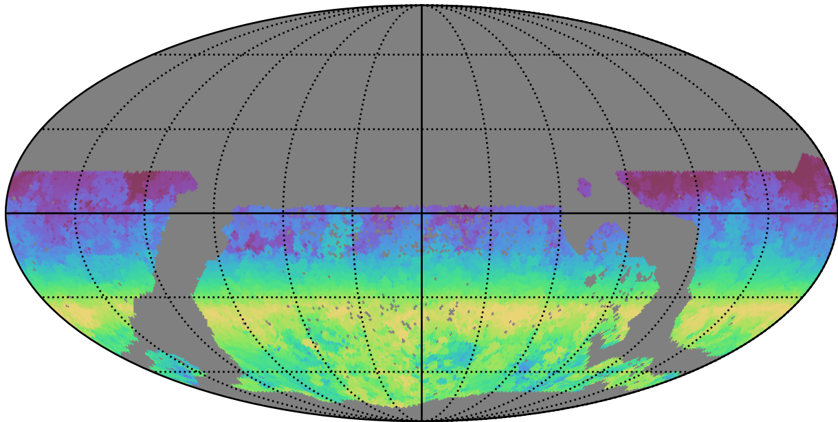
mw_roll_bulge_v3.3_10yrs WFD r band: AngleRange rotSkyPos
