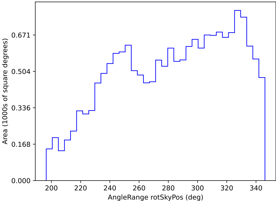
mw_roll_bulge_v3.3_10yrs WFD r band: AngleRange rotSkyPos
