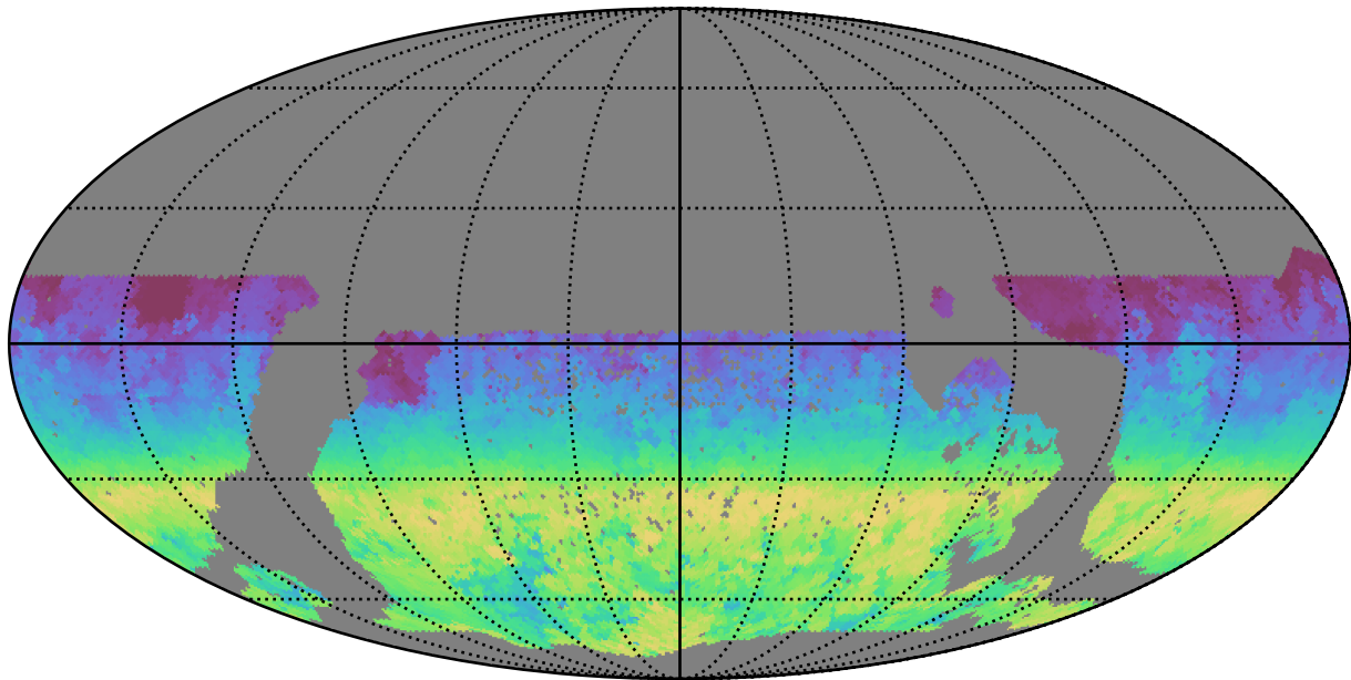
mw_roll_bulge_v3.3_10yrs WFD i band: AngleRange rotSkyPos
