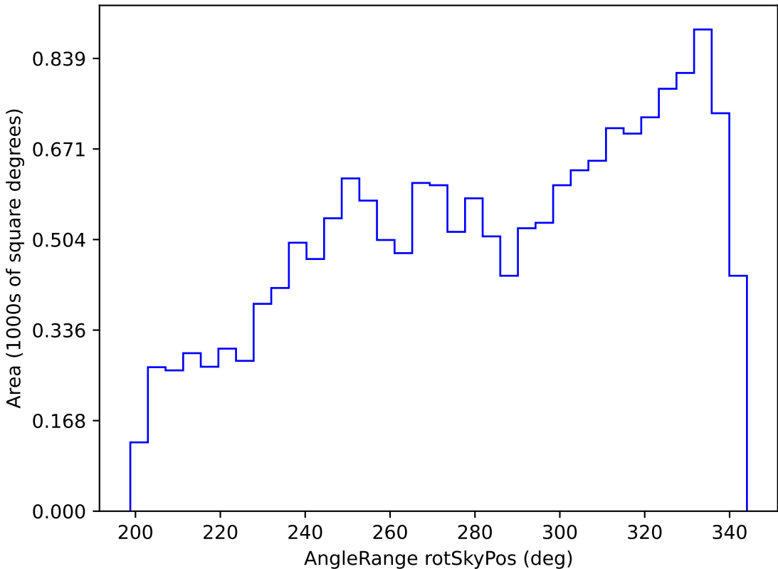
mw_roll_bulge_v3.3_10yrs WFD i band: AngleRange rotSkyPos
