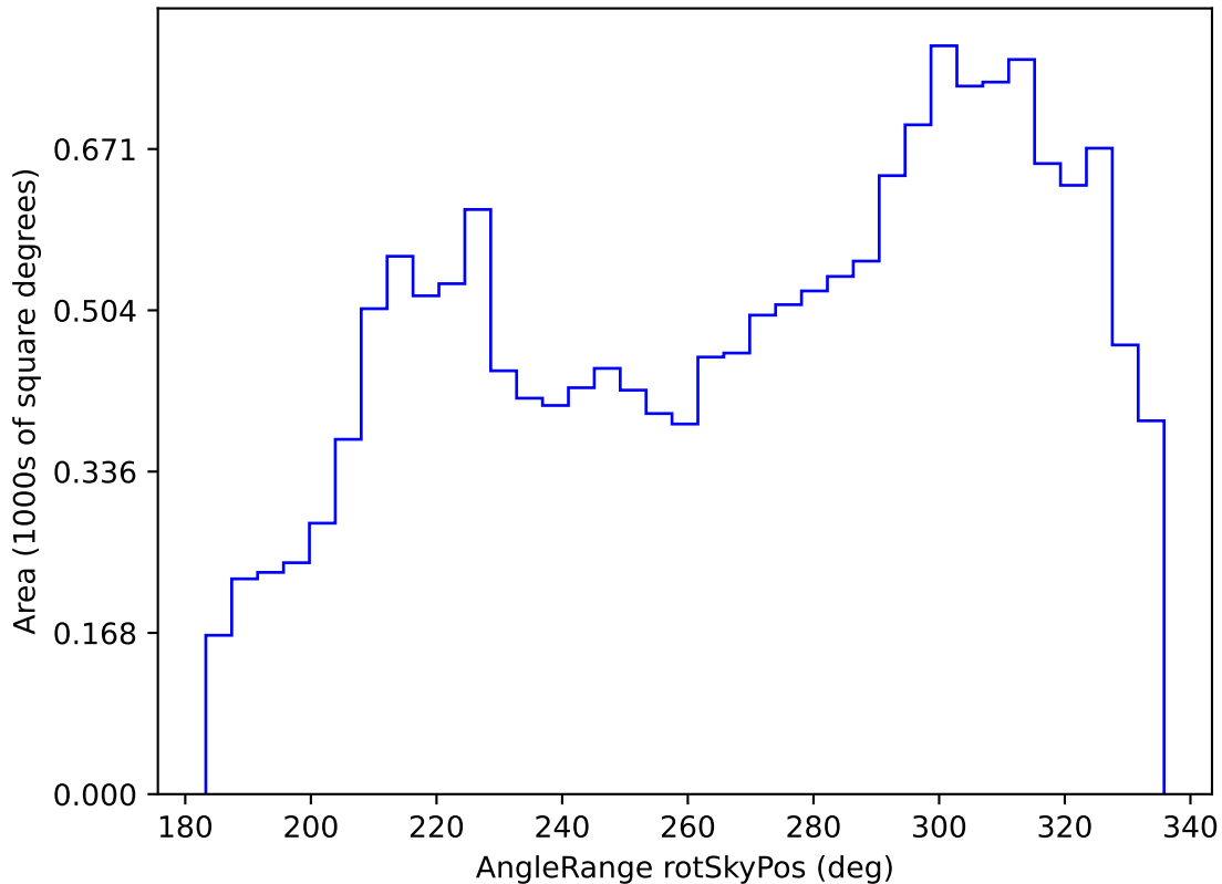
mw_roll_bulge_v3.3_10yrs WFD g band: AngleRange rotSkyPos
