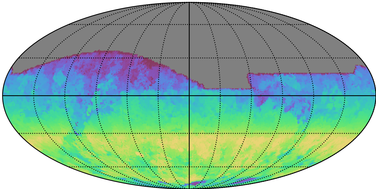
mw_roll_bulge_v3.3_10yrs All sky z band: AngleRange rotSkyPos
