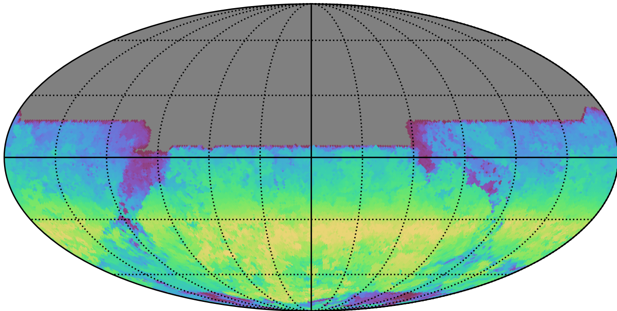
mw_roll_bulge_v3.3_10yrs All sky y band: AngleRange rotSkyPos
