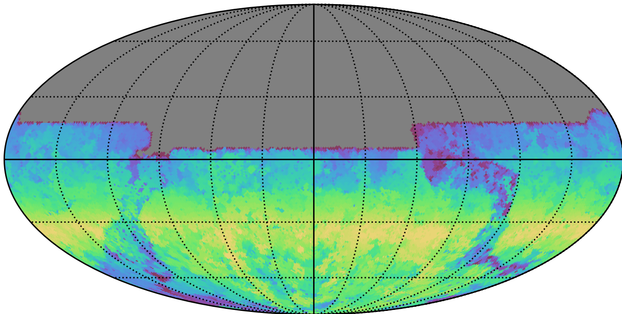
mw_roll_bulge_v3.3_10yrs All sky u band: AngleRange rotSkyPos
