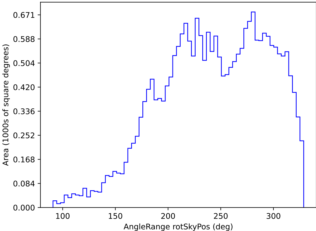
mw_roll_bulge_v3.3_10yrs All sky u band: AngleRange rotSkyPos
