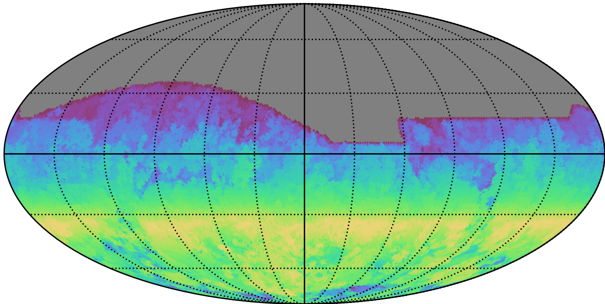
mw_roll_bulge_v3.3_10yrs All sky r band: AngleRange rotSkyPos
