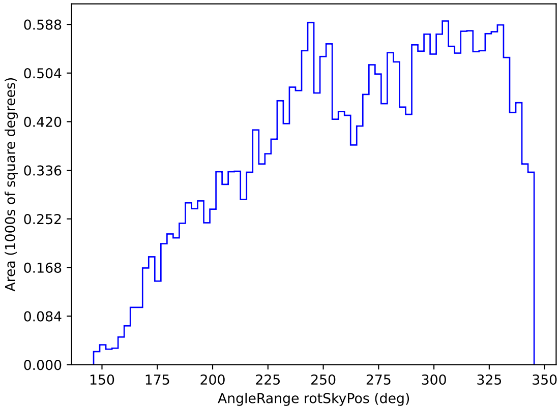
mw_roll_bulge_v3.3_10yrs All sky r band: AngleRange rotSkyPos
