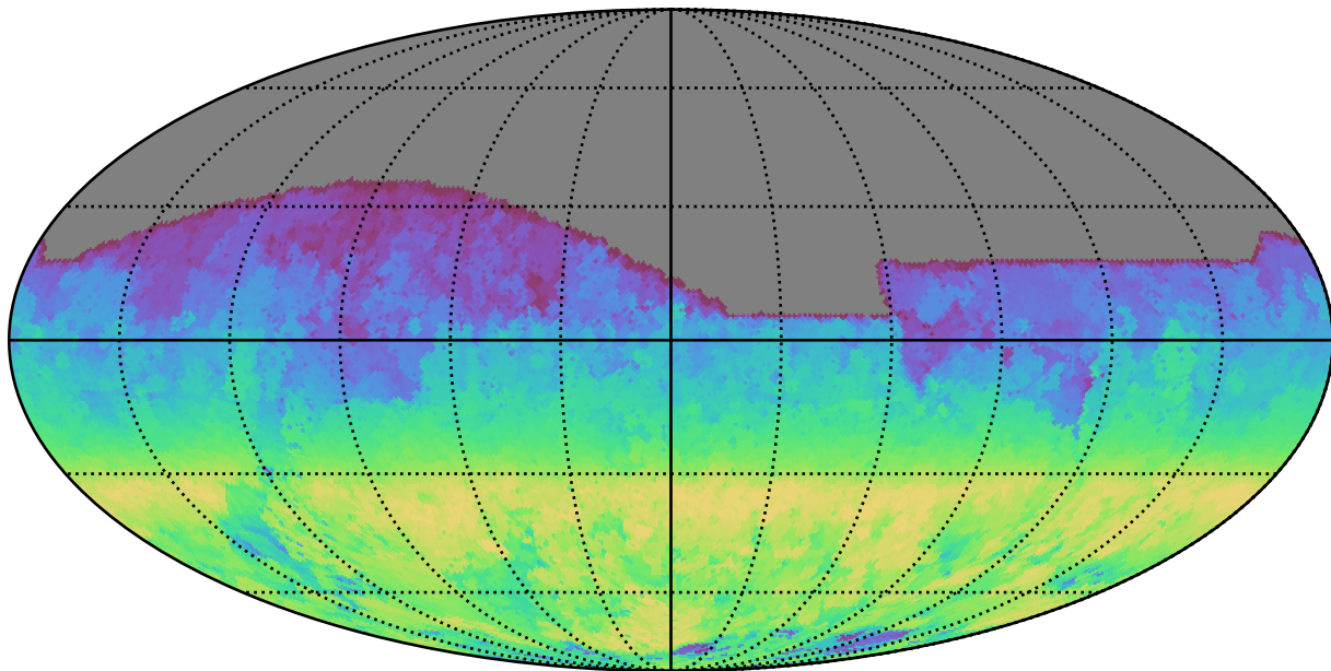
mw_roll_bulge_v3.3_10yrs All sky i band: AngleRange rotSkyPos
