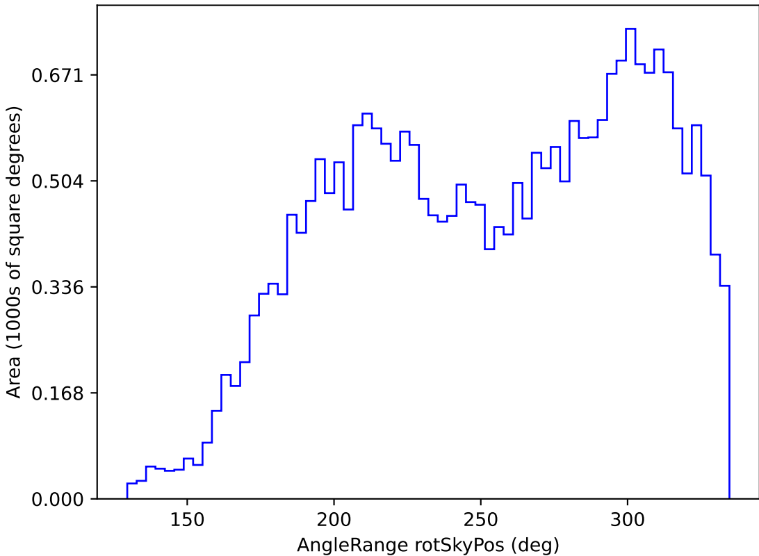
mw_roll_bulge_v3.3_10yrs All sky g band: AngleRange rotSkyPos
