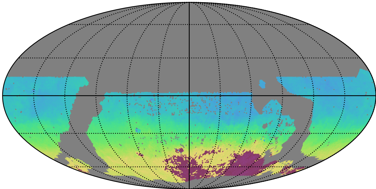
mw_roll_bulge_v3.3_10yrs WFD y band: AngleMean rotSkyPos
