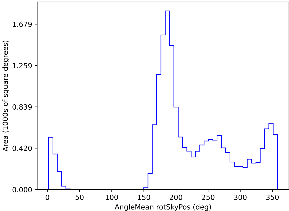
mw_roll_bulge_v3.3_10yrs WFD y band: AngleMean rotSkyPos
