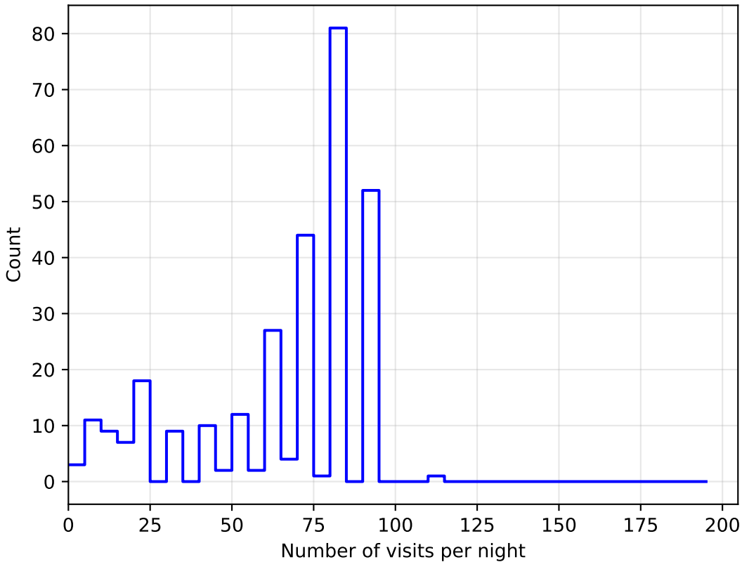
mw_roll_bulge_v3.3_10yrs all bands: DD:ELAISS1 NVisitsPerNight
