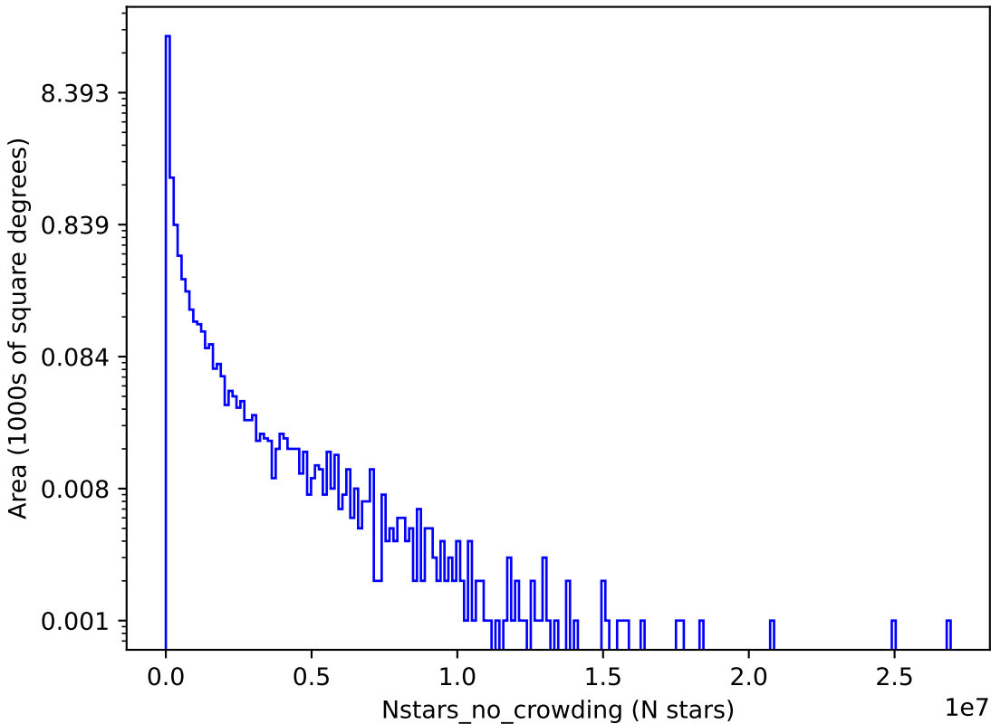
mw_roll_all_v3.3_10yrs z: Nstars_no_crowding
