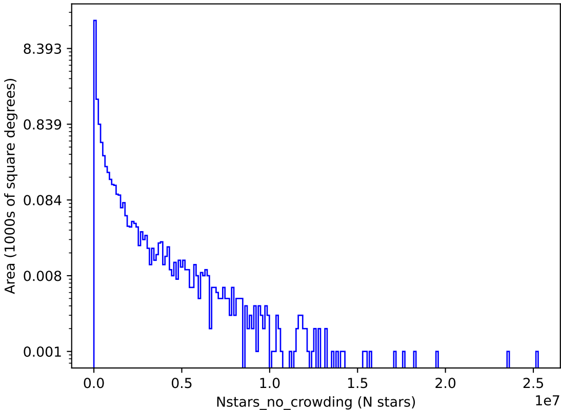
mw_roll_all_v3.3_10yrs y: Nstars_no_crowding
