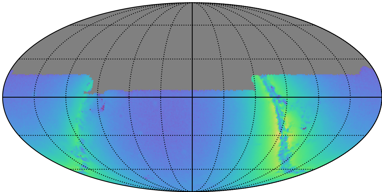
mw_roll_all_v3.3_10yrs u: Nstars_no_crowding
