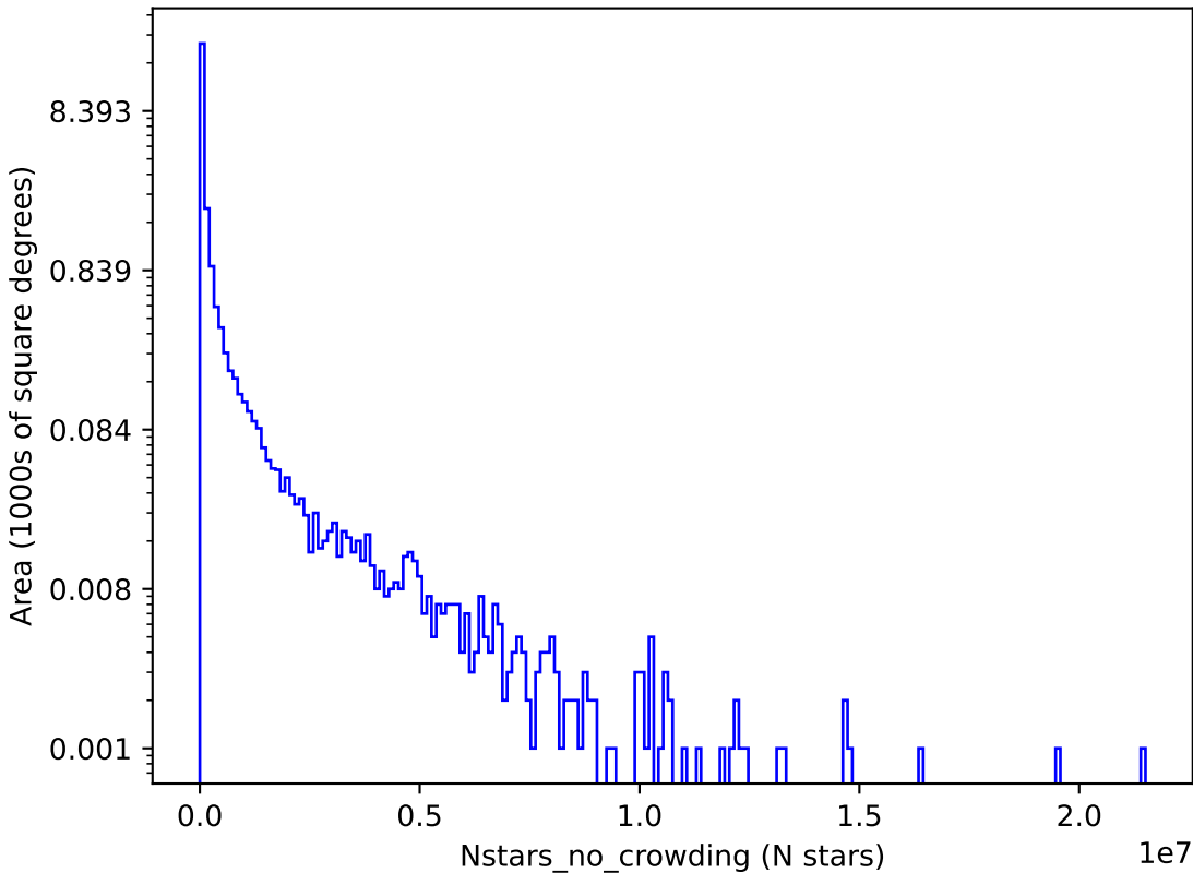
mw_roll_all_v3.3_10yrs r: Nstars_no_crowding
