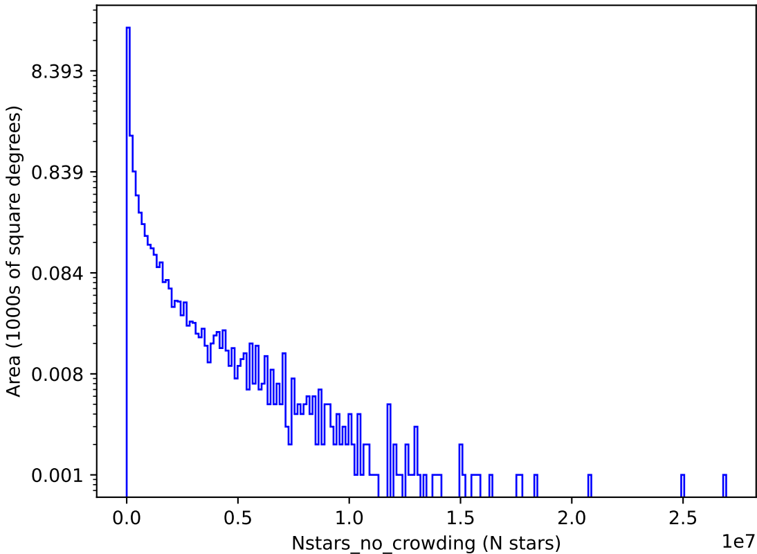
mw_roll_all_v3.3_10yrs i: Nstars_no_crowding
