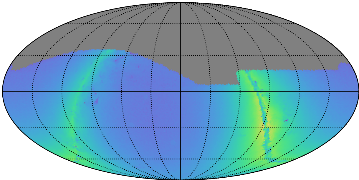
mw_roll_all_v3.3_10yrs g: Nstars_no_crowding
