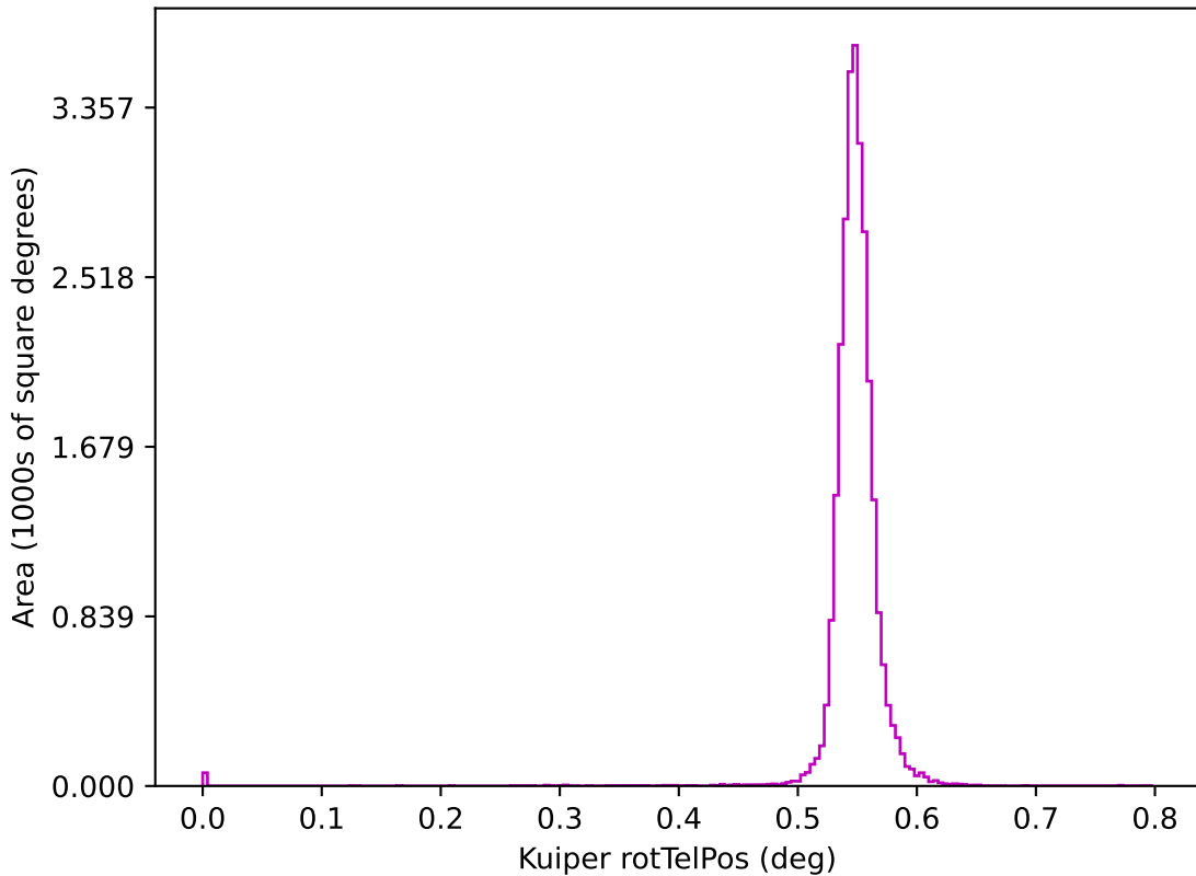
mw_roll_all_v3.3_10yrs z: Kuiper rotTelPos
