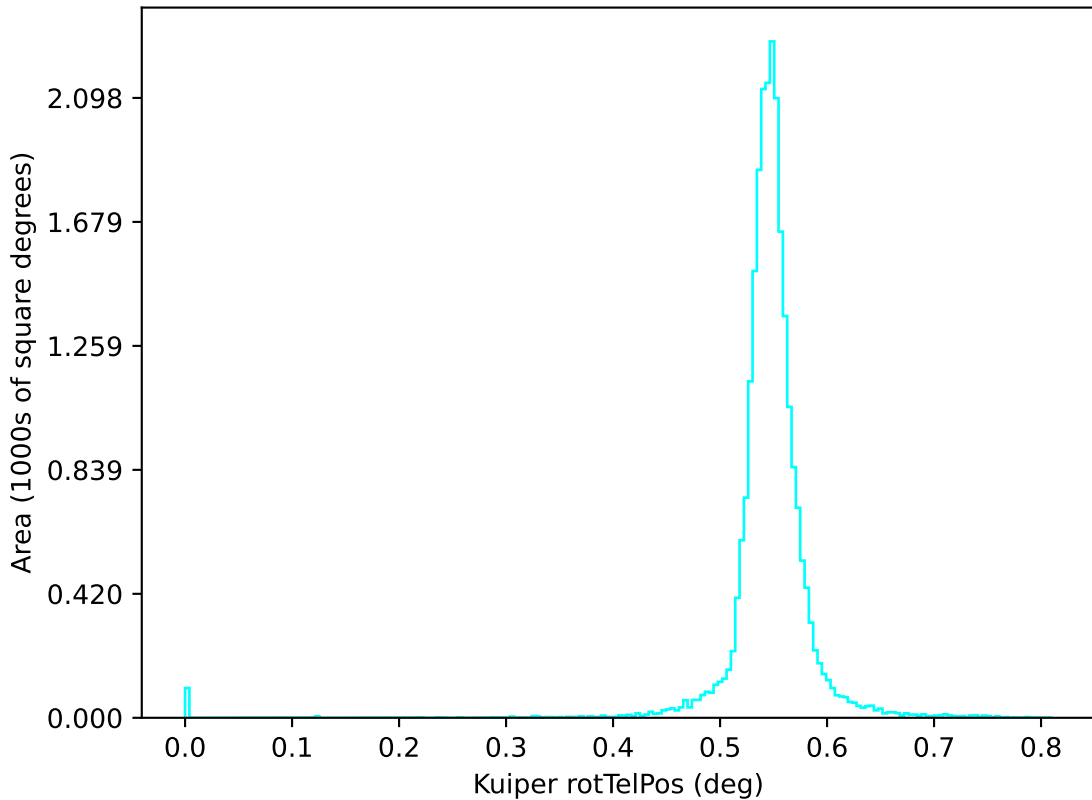
mw_roll_all_v3.3_10yrs u: Kuiper rotTelPos
