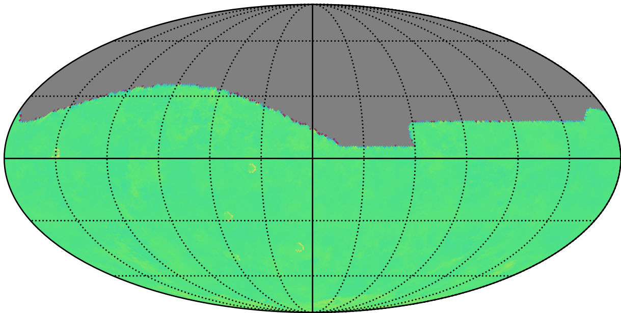
mw_roll_all_v3.3_10yrs r: Kuiper rotTelPos
