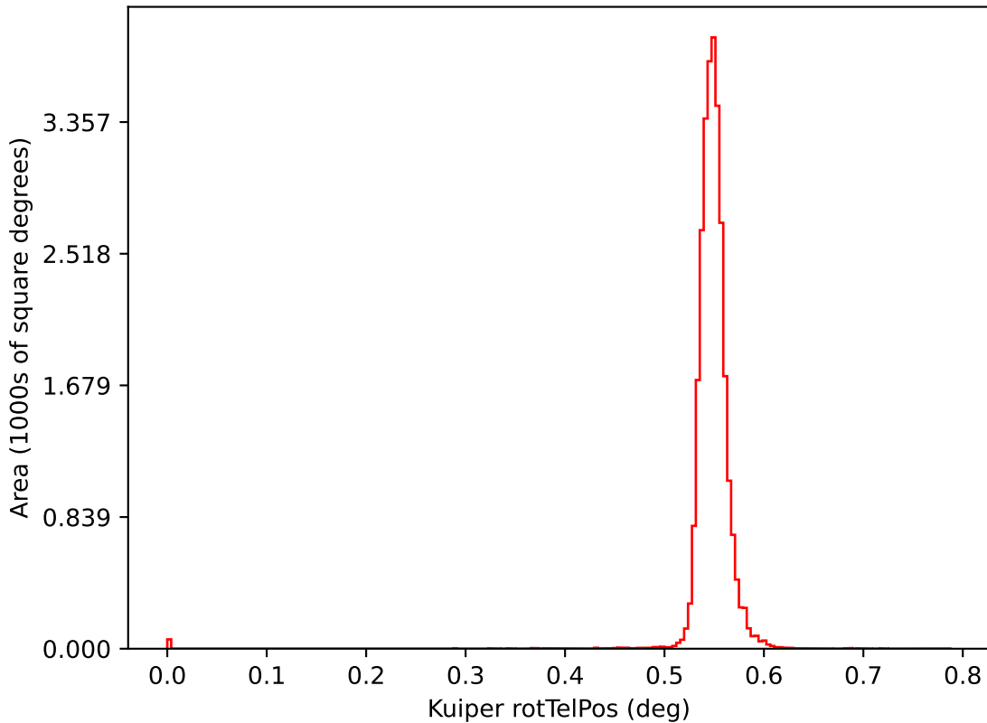
mw_roll_all_v3.3_10yrs i: Kuiper rotTelPos
