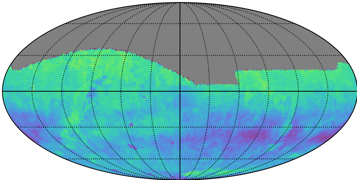
mw_roll_all_v3.3_10yrs z: Kuiper rotSkyPos
