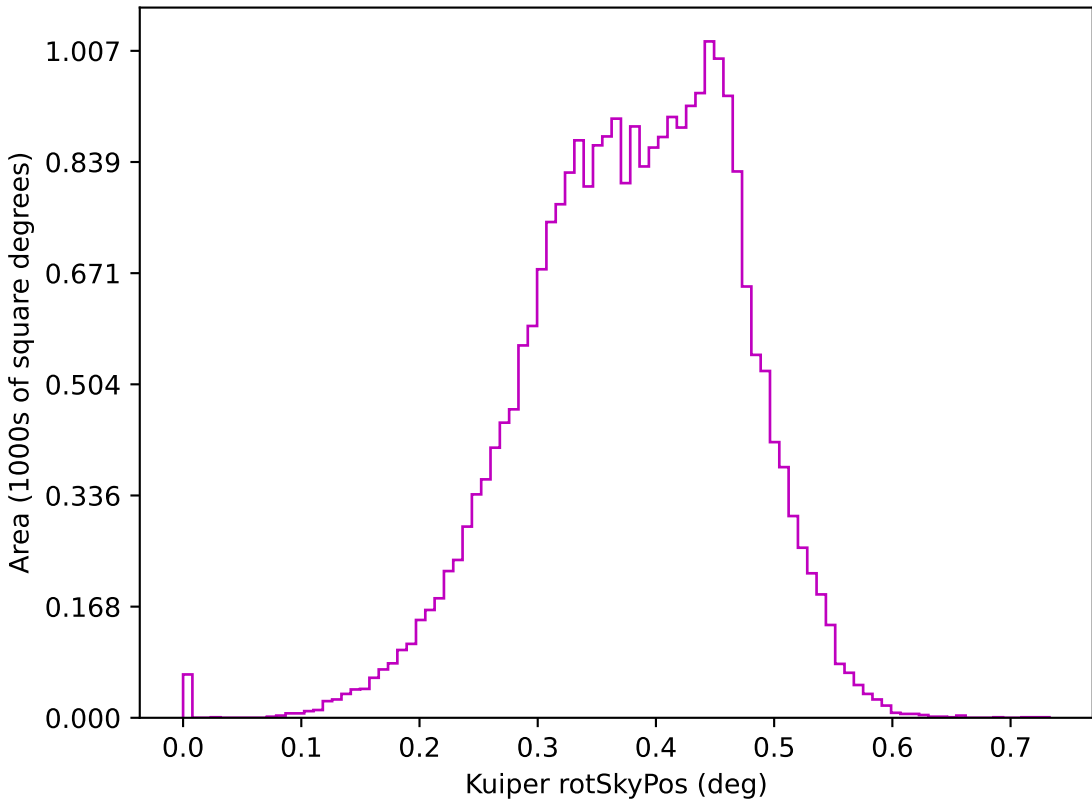
mw_roll_all_v3.3_10yrs z: Kuiper rotSkyPos
