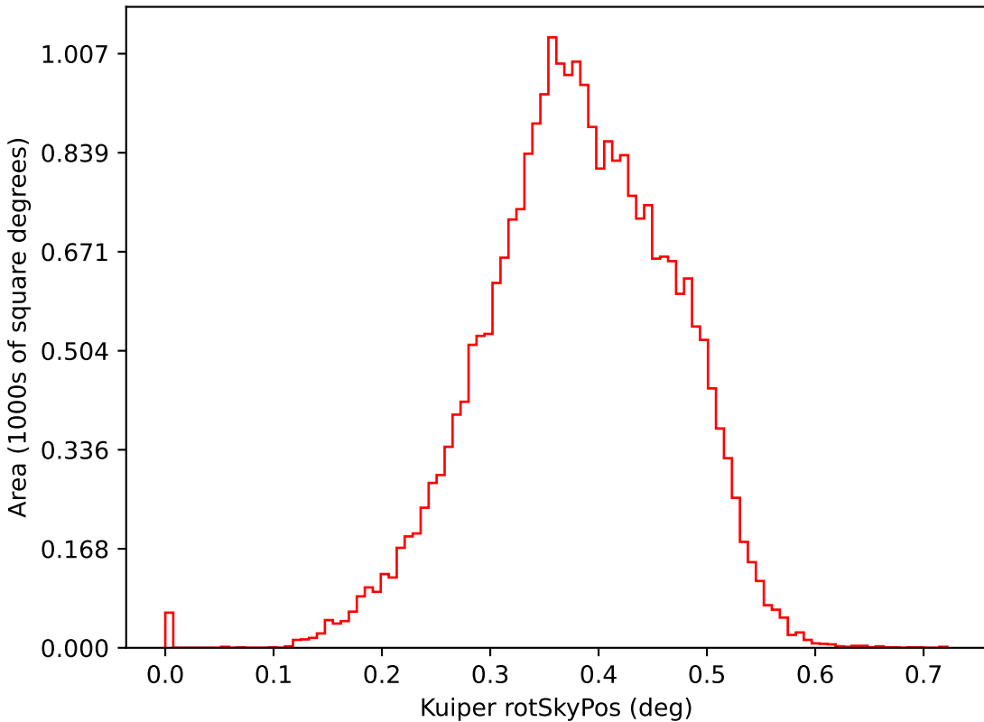
mw_roll_all_v3.3_10yrs i: Kuiper rotSkyPos
