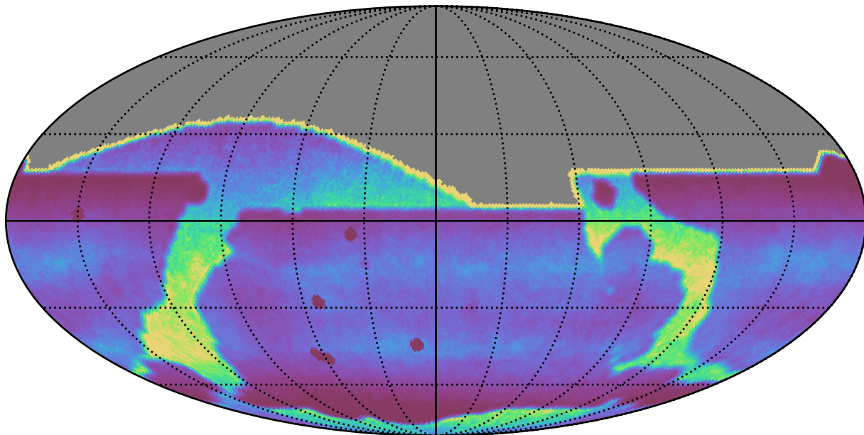
mw_roll_all_v3.3_10yrs : DCRprecision
