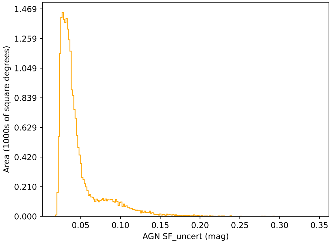
mw_roll_all_v3.3_10yrs r band: AGN SF_uncert
