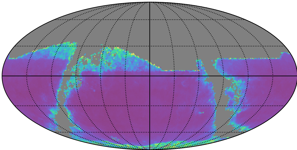
mw_roll_all_v3.3_10yrs i band: AGN SF_uncert
