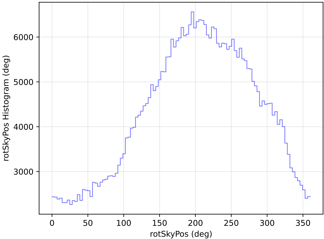
mw_roll_all_v3.3_10yrs WFD z band: rotSkyPos Histogram
