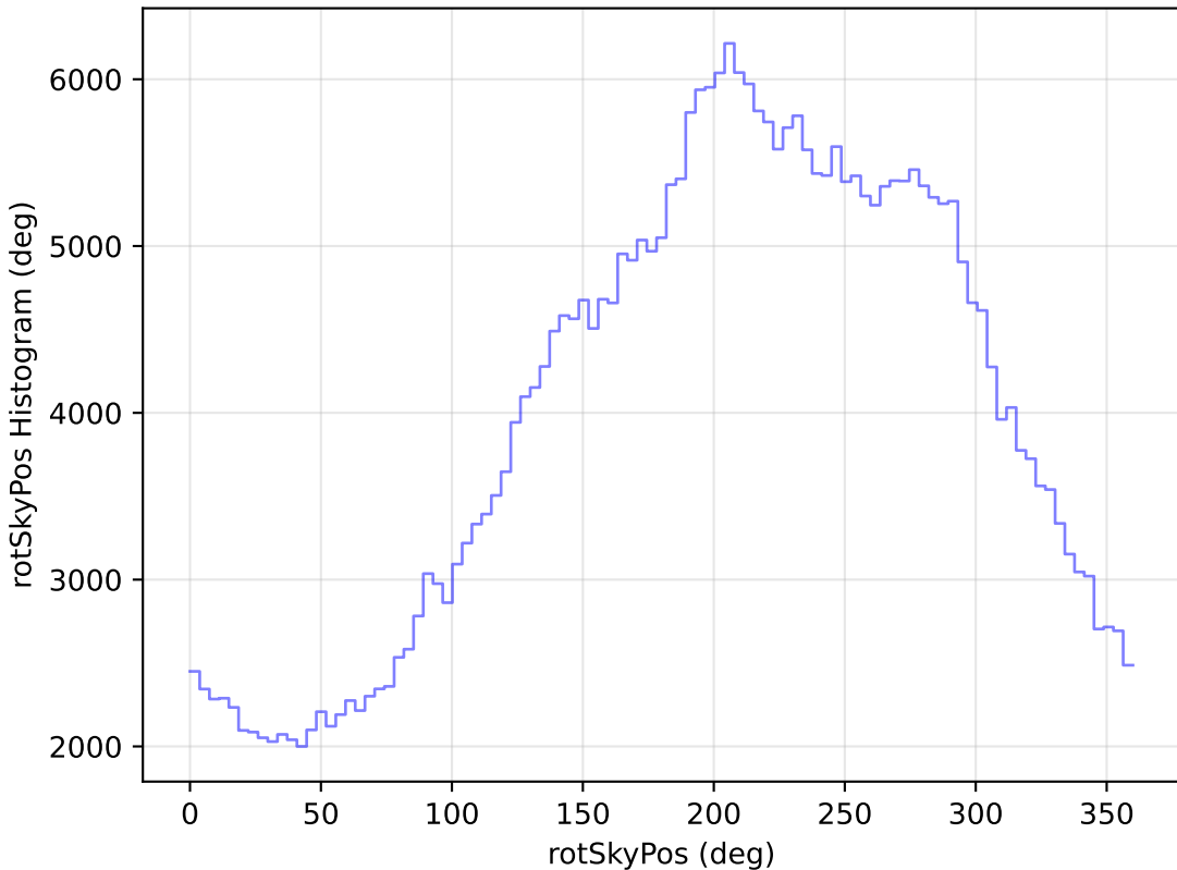
mw_roll_all_v3.3_10yrs WFD y band: rotSkyPos Histogram
