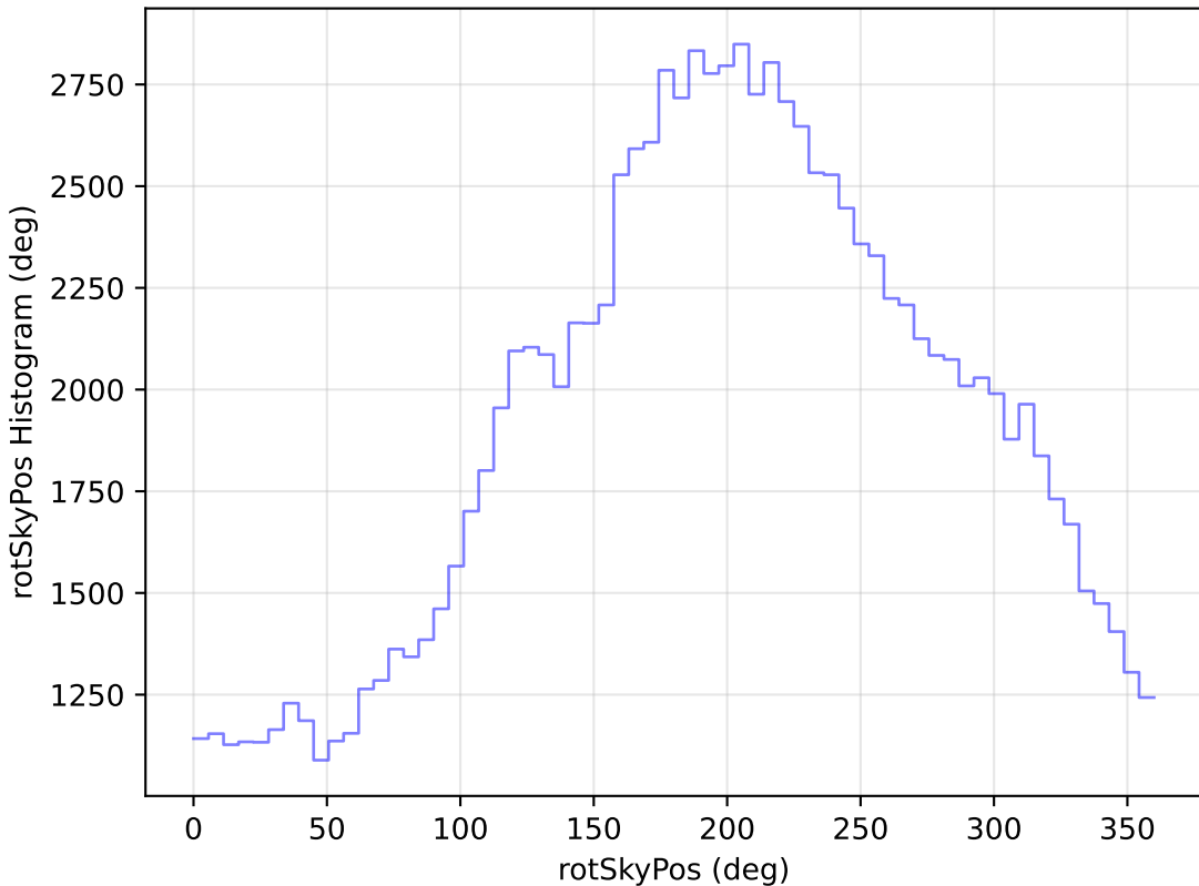
mw_roll_all_v3.3_10yrs WFD u band: rotSkyPos Histogram
