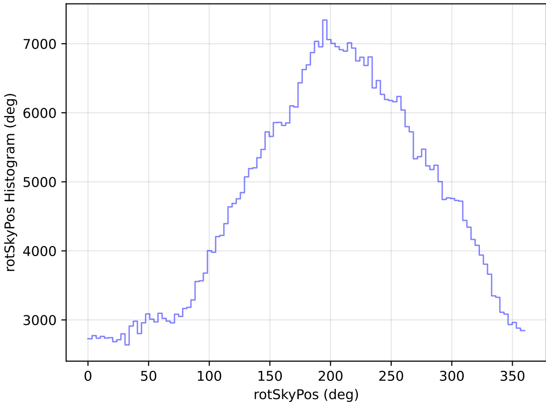
mw_roll_all_v3.3_10yrs WFD i band: rotSkyPos Histogram
