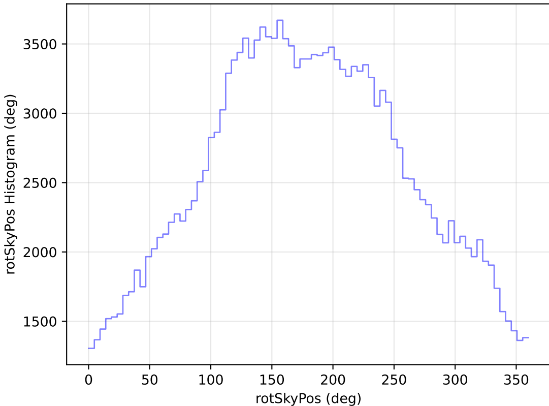
mw_roll_all_v3.3_10yrs WFD g band: rotSkyPos Histogram
