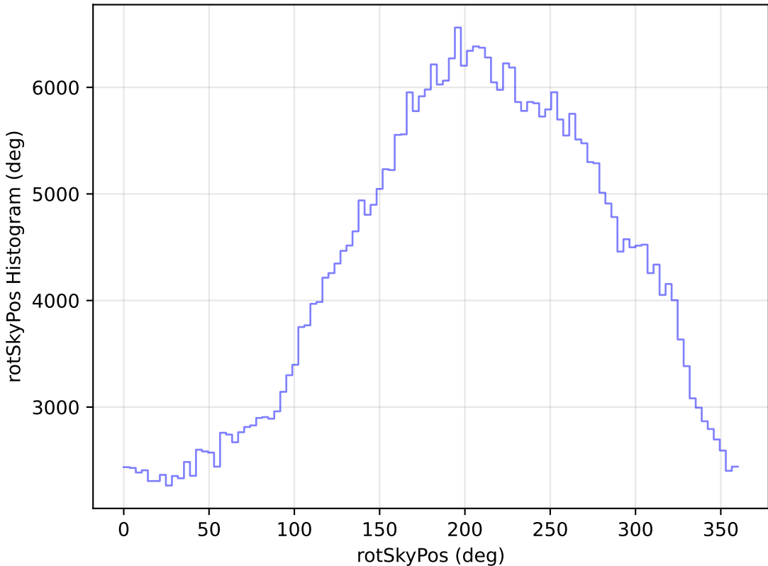
mw_roll_all_v3.3_10yrs All sky z band: rotSkyPos Histogram
