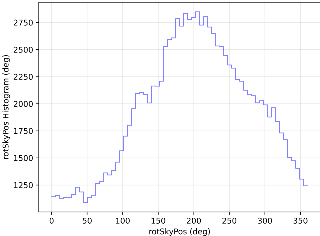
mw_roll_all_v3.3_10yrs All sky u band: rotSkyPos Histogram
