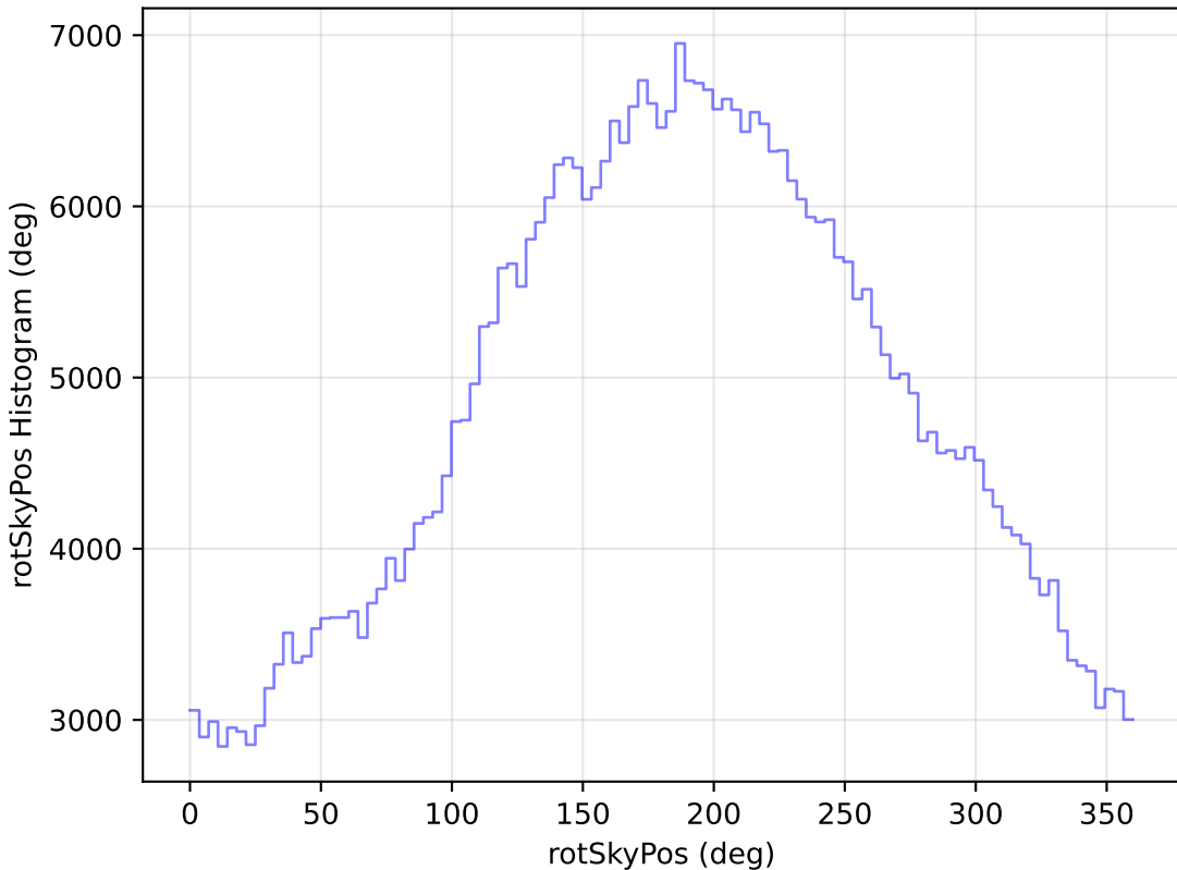
mw_roll_all_v3.3_10yrs All sky r band: rotSkyPos Histogram
