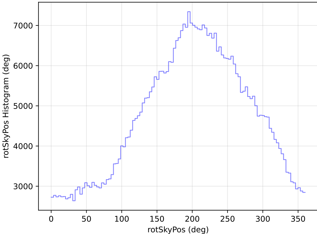
mw_roll_all_v3.3_10yrs All sky i band: rotSkyPos Histogram
