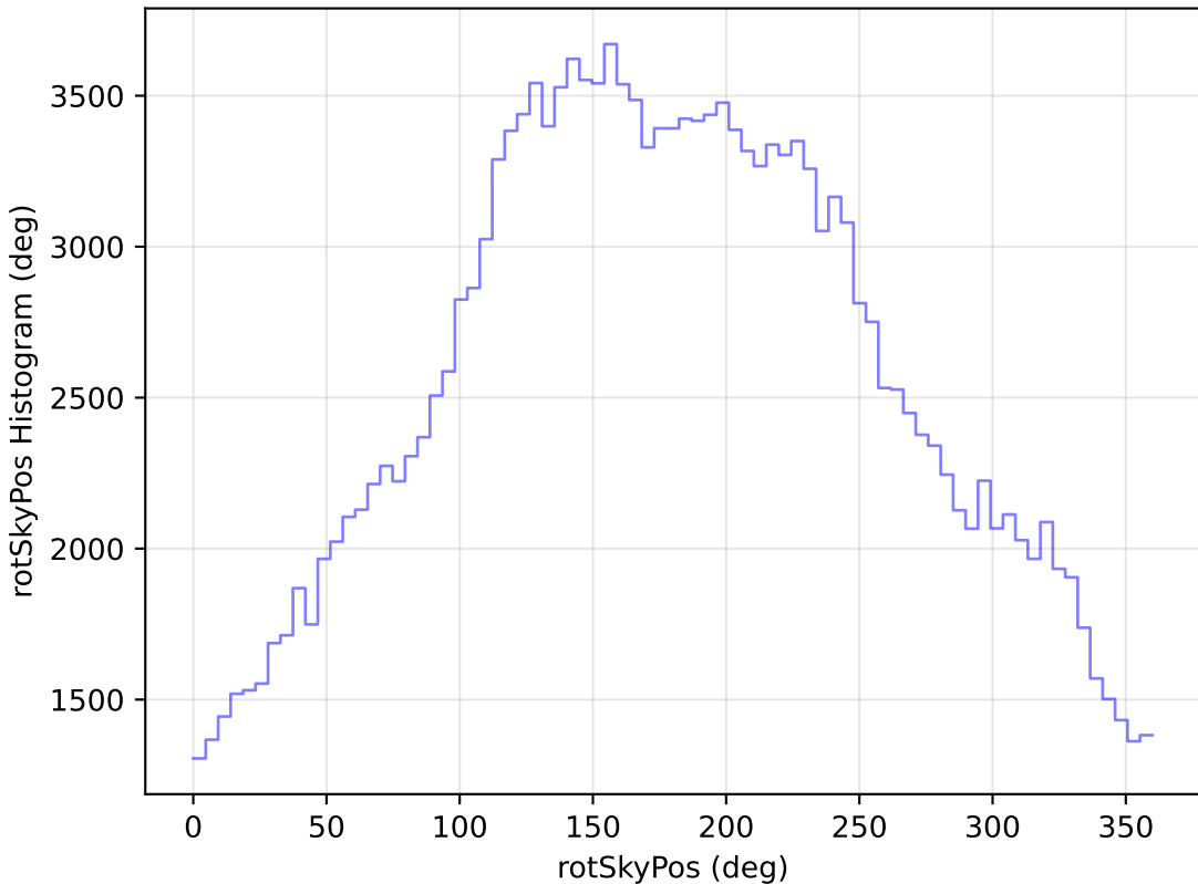
mw_roll_all_v3.3_10yrs All sky g band: rotSkyPos Histogram
