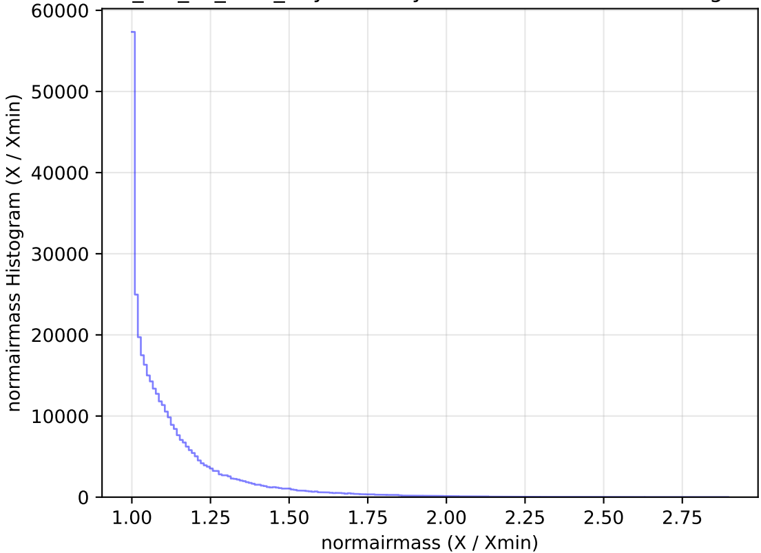
mw_roll_all_v3.3_10yrs WFD y band: normairmass Histogram
