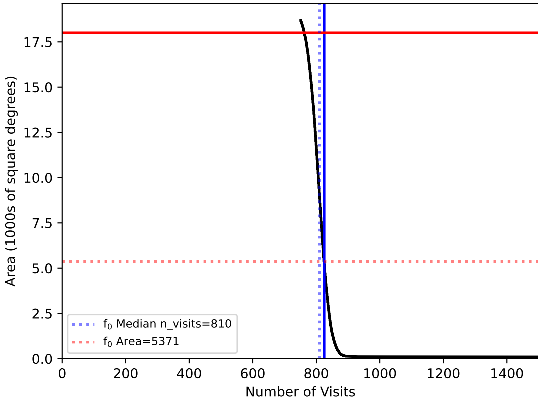
mw_roll_all_v3.3_10yrs WFD: f0
