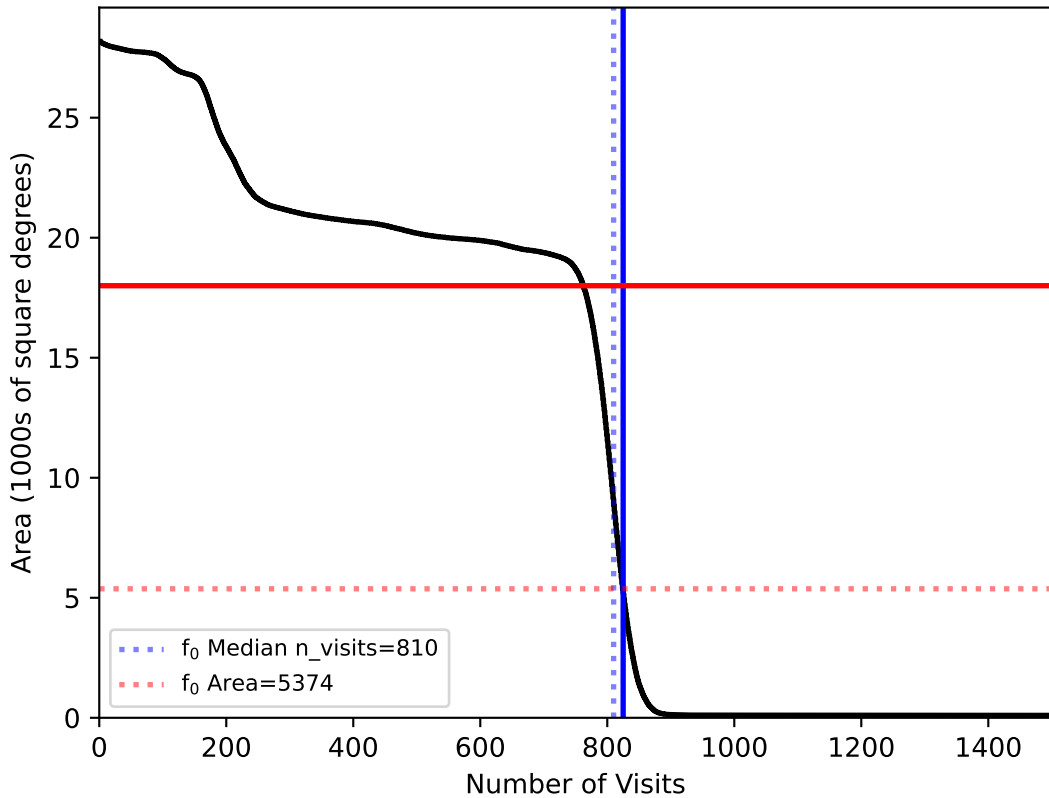
mw_roll_all_v3.3_10yrs All sky: f0
