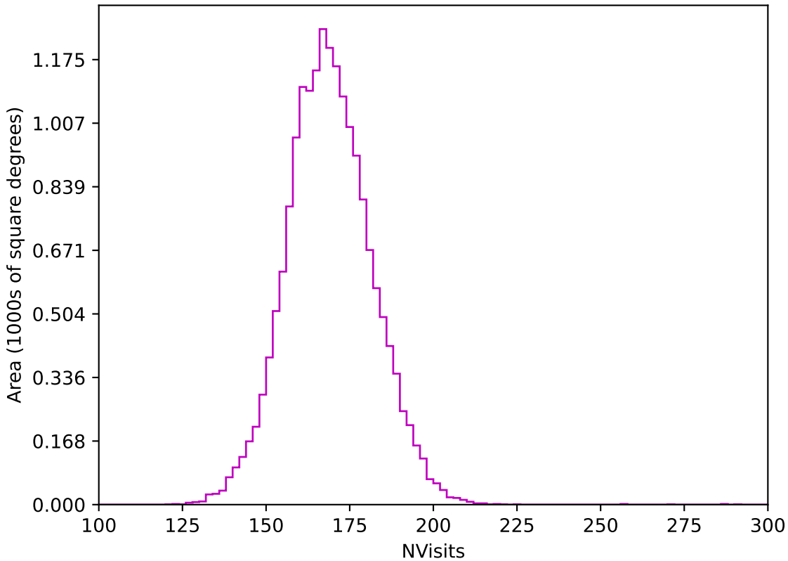
mw_roll_all_v3.3_10yrs WFD z band: NVisits
