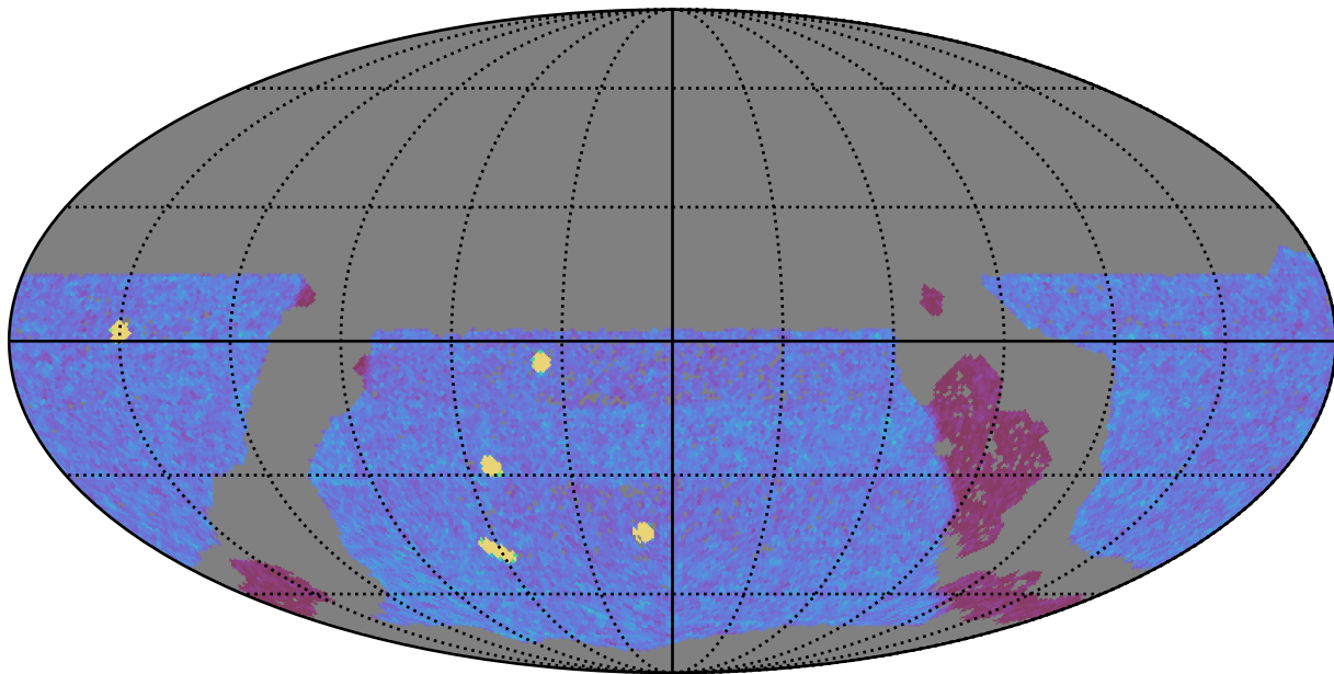
mw_roll_all_v3.3_10yrs WFD y band: NVisits
