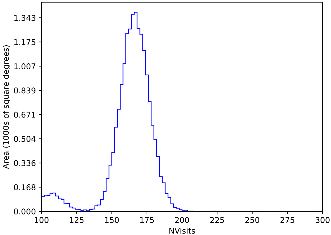
mw_roll_all_v3.3_10yrs WFD y band: NVisits
