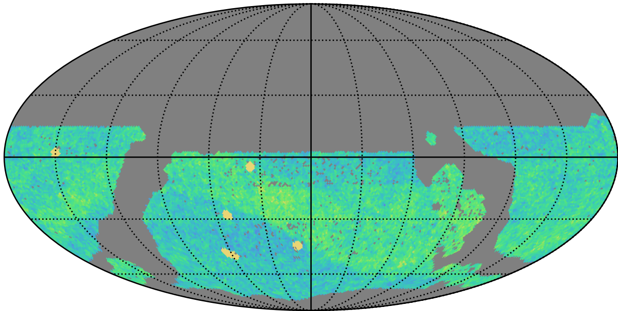
mw_roll_all_v3.3_10yrs WFD i band: NVisits
