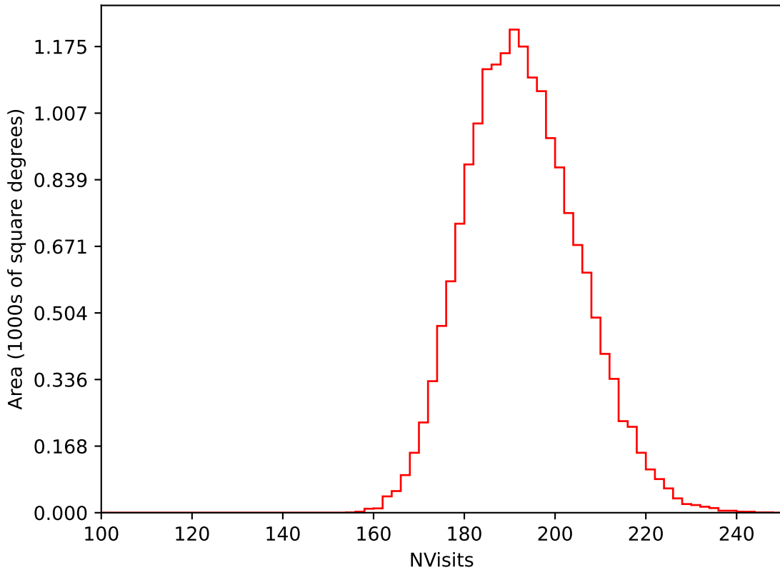
mw_roll_all_v3.3_10yrs WFD i band: NVisits
